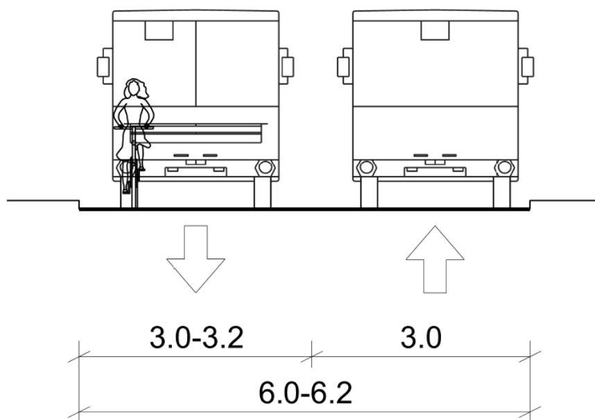
Rys. 22 Przykład rozwiązania przekroju jezdni autobusowej wykorzystywanej wspólnie przez ruch rowerowy i autobusowy. Przy szerokości pasa autobusowo-rowerowego 3.0-3.2m.
