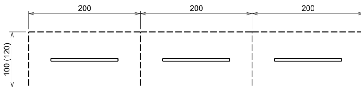
Rys. 45 Schemat równoległego usytuowania miejsc do parkowania rowerów.
