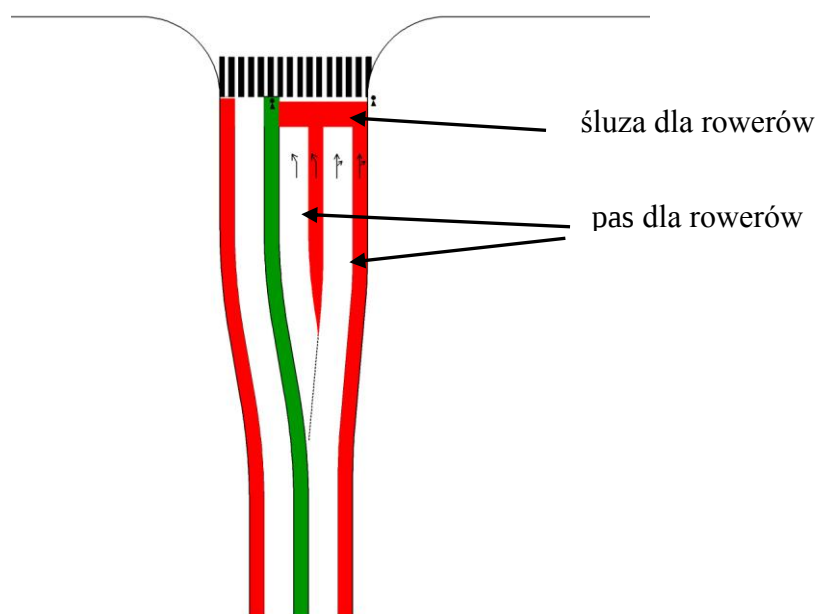
Rys. 21 Przykład rozwiązania wlotu na skrzyżowanie z ruchem rowerowym prowadzonym w jezdni, z zastosowaniem śluzy dla ruchu rowerowego i wydzielonych pasów do skrętu w lewo.
