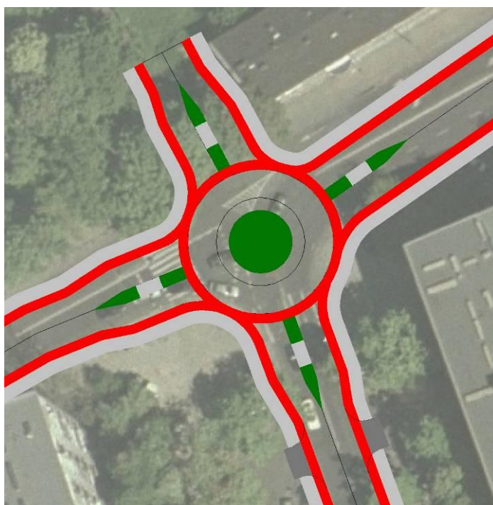
Rys. 17 Schemat rozwiązania ronda położonego poza strefą o ruchu uspokojonym z ruchem rowerowym prowadzonym po obwodnicy.
