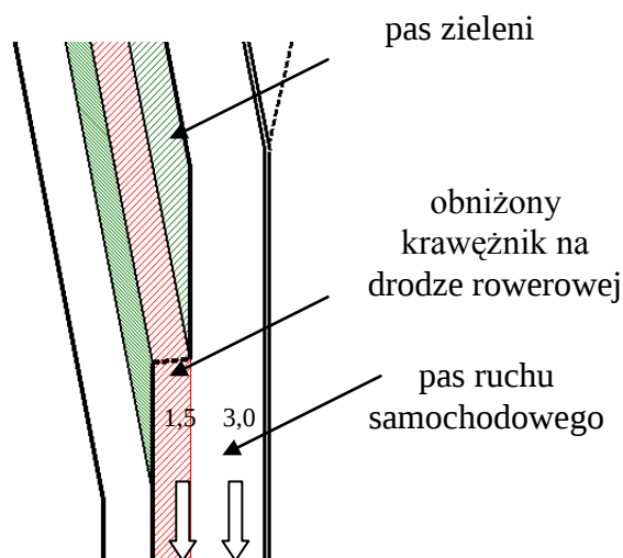
Rys. 14 Wjazd na ścieżkę rowerową stanowiącą kontynuację pasa dla rowerów (z krawężnikiem wystającym na styku obu dróg dla rowerów, nie większym niż 1 cm).
