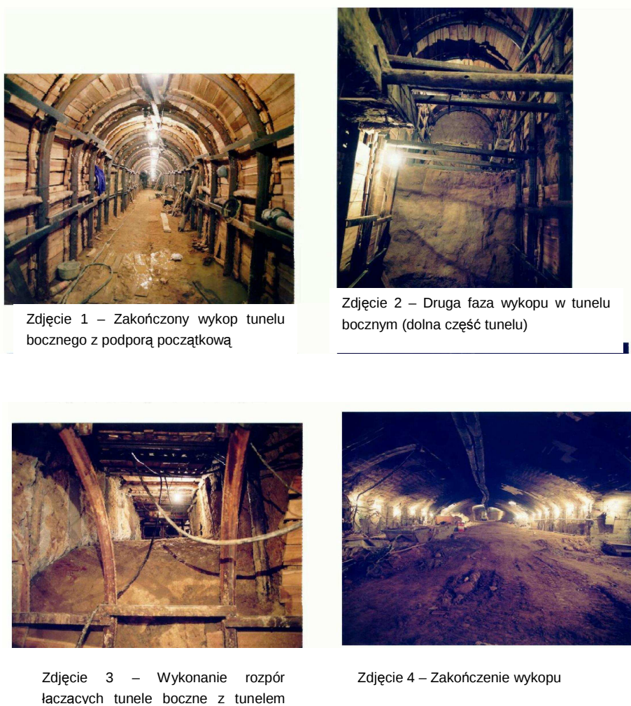
Rysunek 2. 15 Przykłady etapów budowy do wykonania wykopu metodą niemiecką
