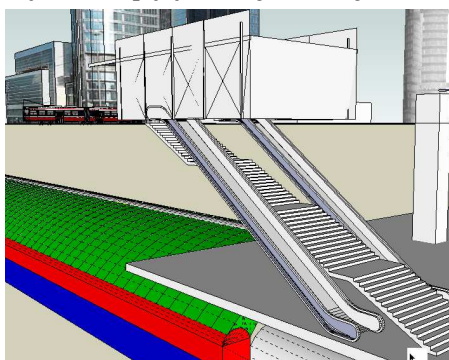
Rysunek 2. 11 Wykonanie płyty dennej oraz wejść do stacji metra
