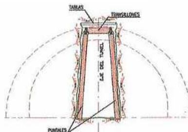
Rysunek 2. 16 Etapy budowy metodą belgijską
