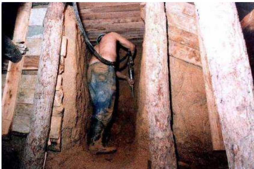
Rysunek 2. 17 Przykładowa budowa tunelu metoda belgijską: powiększanie tunelu
