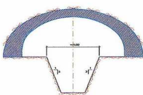
4. Dalsze wykonanie tunelu – wykop w galerii.
